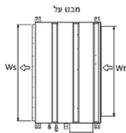
מידות פתחי אספקה ואוויר חוזר ליחידות מתועלות
